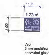
S.W. Elevation
