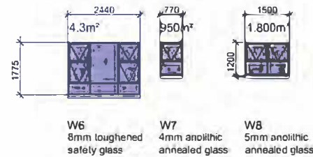
N.W. Elevation
