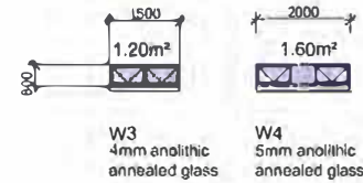
N.W. Elevation
